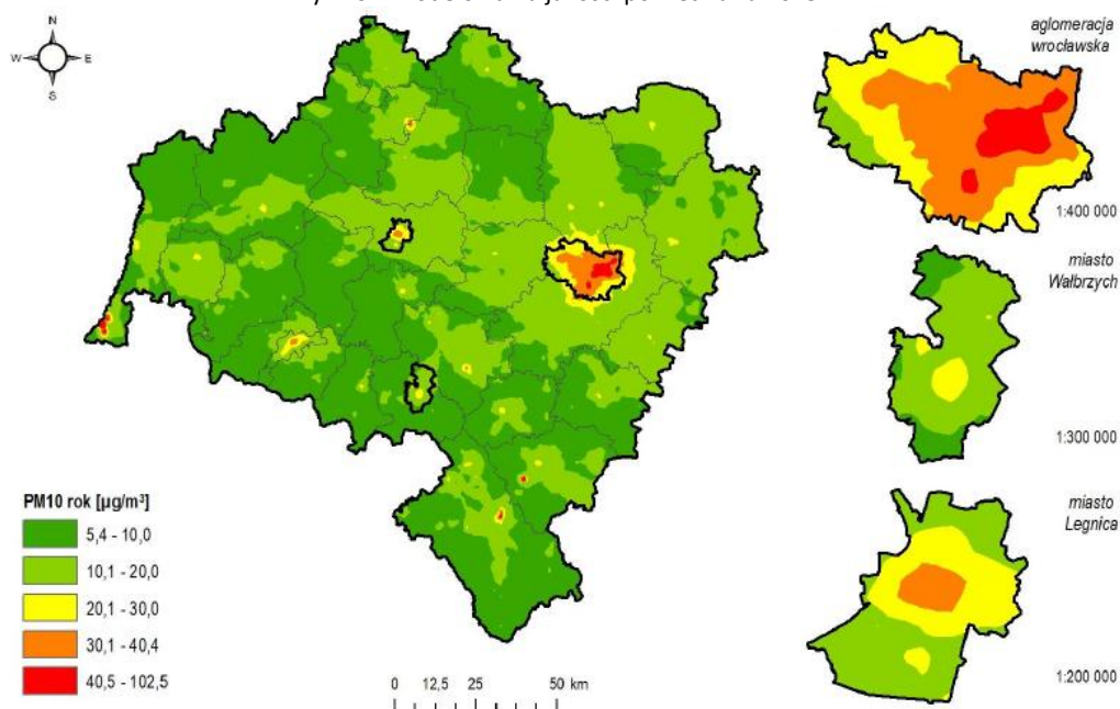
Rysunek 15. Rozkład stężeń średniorocznych pyłu zawieszonego PM 10 na terenie woj. Dolnośląskiego na podstawie wyników modelowania jakości powietrza za 2015.
