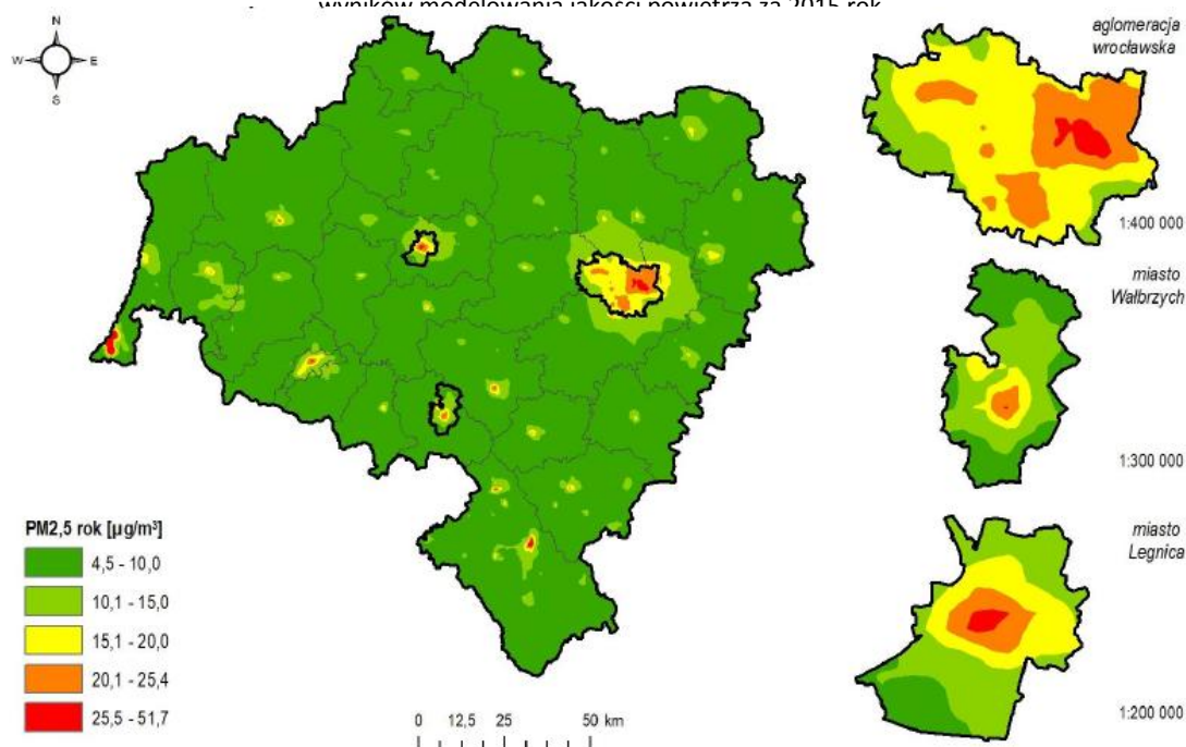
Rysunek 16. Rozkład stężeń średniorocznych pyłu zawieszonego PM2.5 na terenie woj. Dolnośląskiego na podstawie wyników modelowania jakości powietrza za 2015 rok
